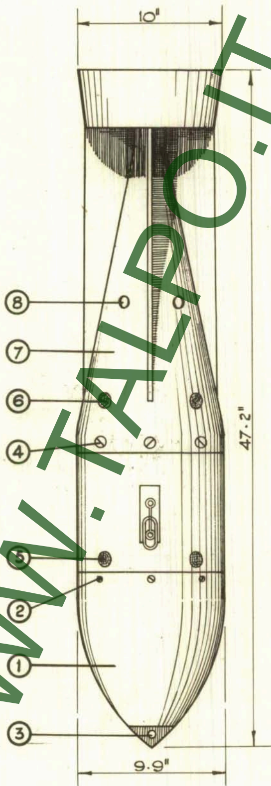
BOMBA 70. I. P.
